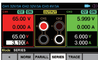
▲ 串联模式图
